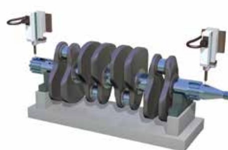
⑥ 工件高度检测
