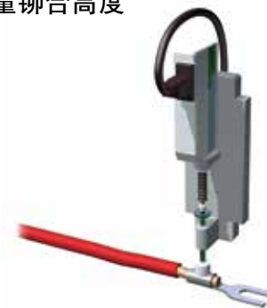
⑤ 测量铆合高度
